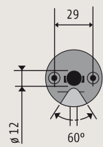
Querschnitt
