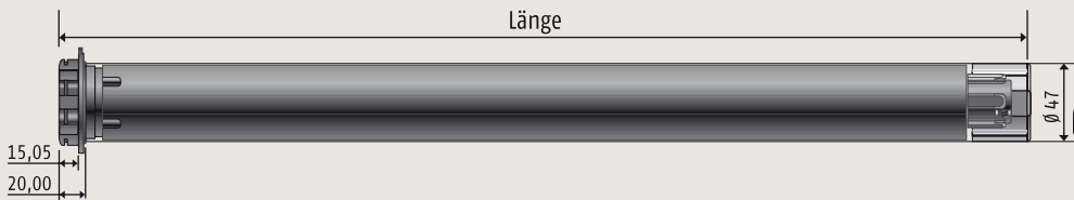
Seitenansicht
