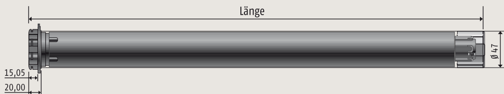
Seitenansicht
